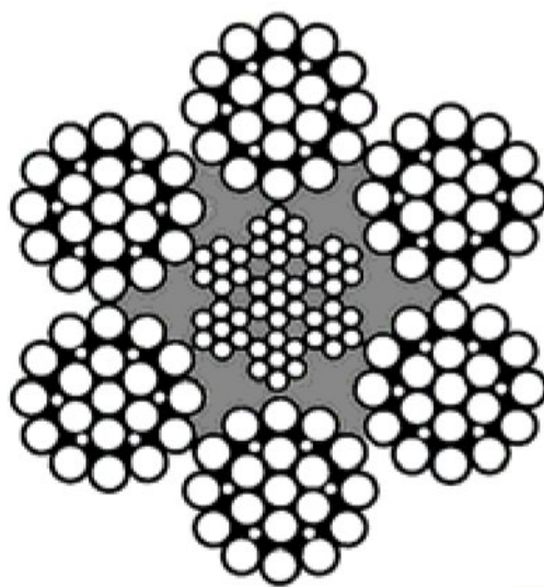
6 x 25 Filler Wire IWRC
