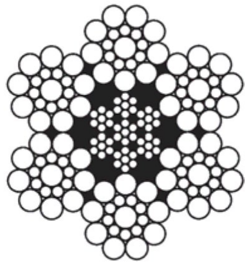
6 x 19 Seale IWRC
