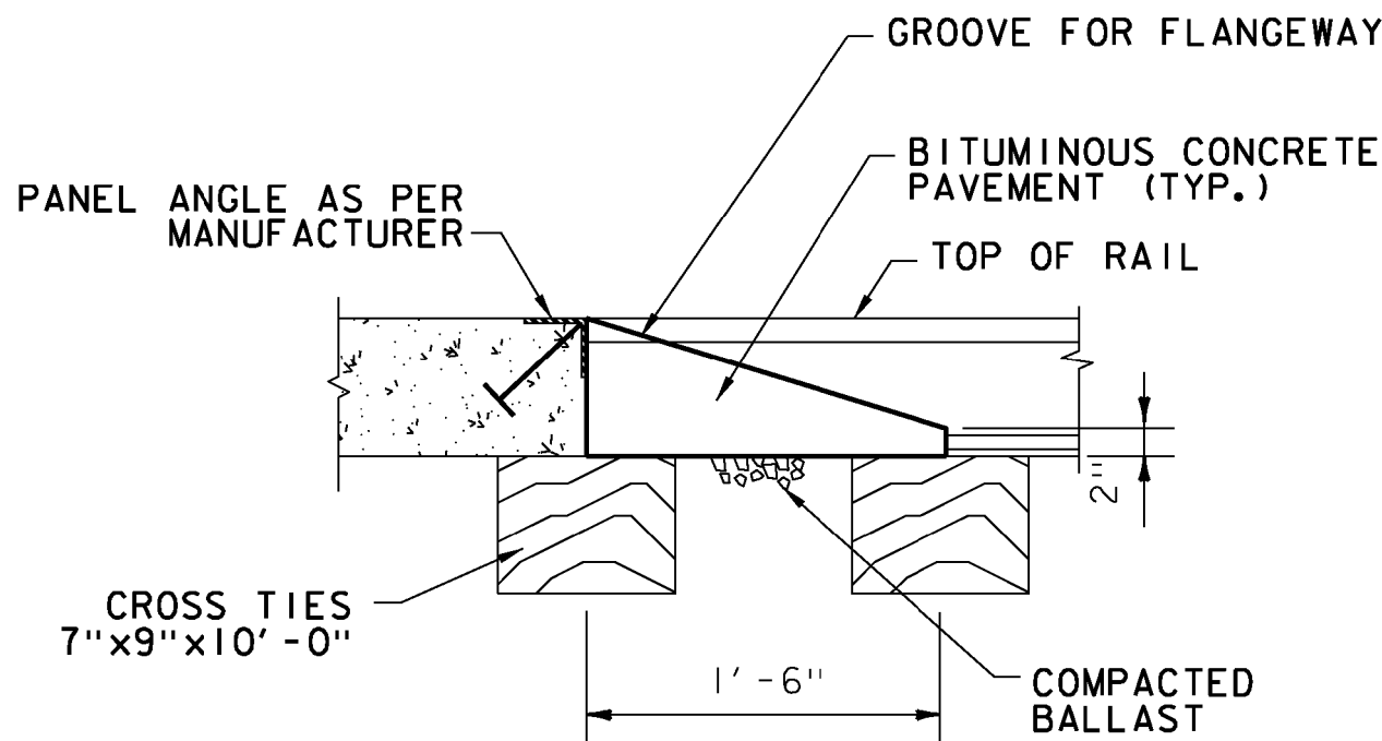
PANEL END SIDE VIEW N. T. S.
