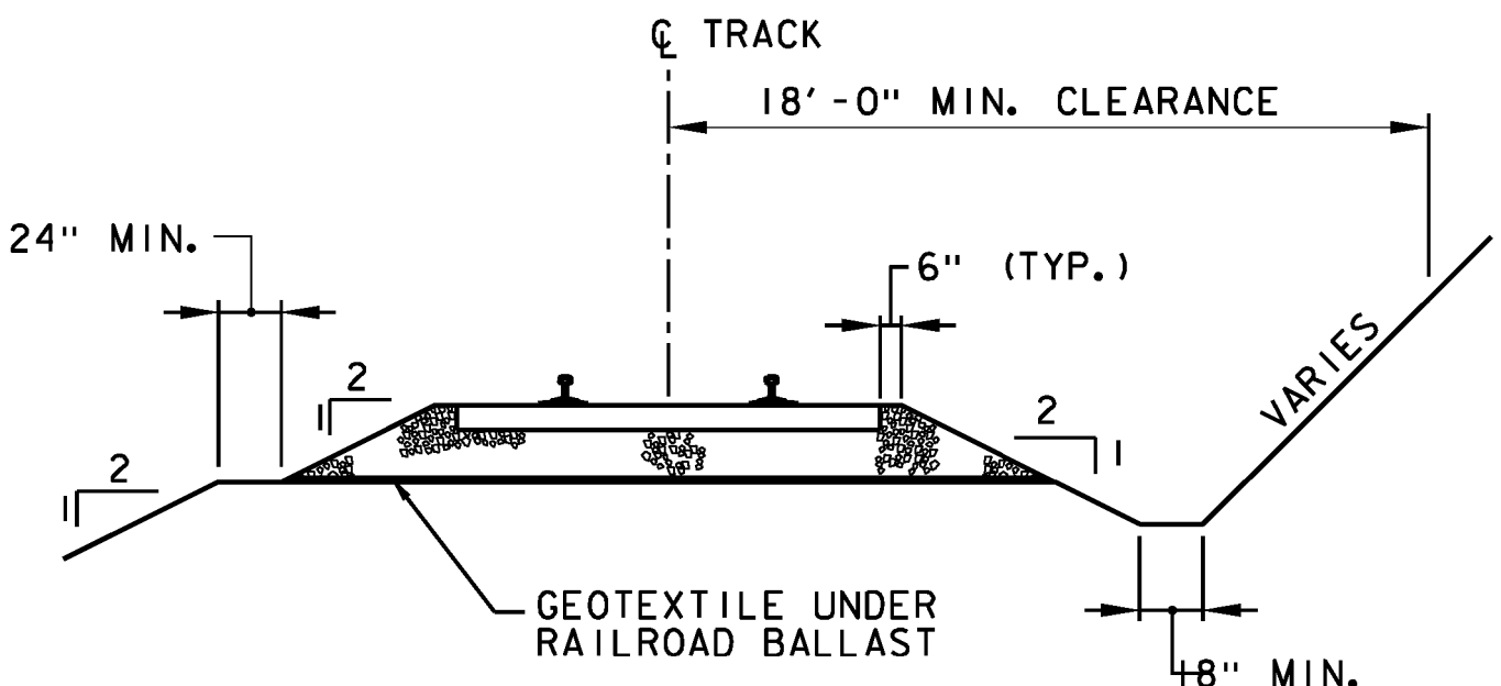
TYPICAL RAIL SECTION N. T. S.
