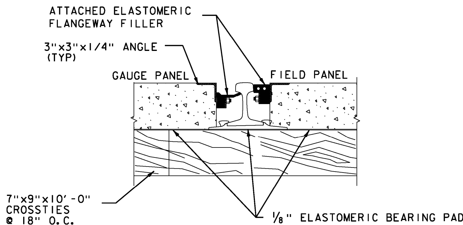
RAIL-SEALS TYPICAL SECTION N. T. S.
