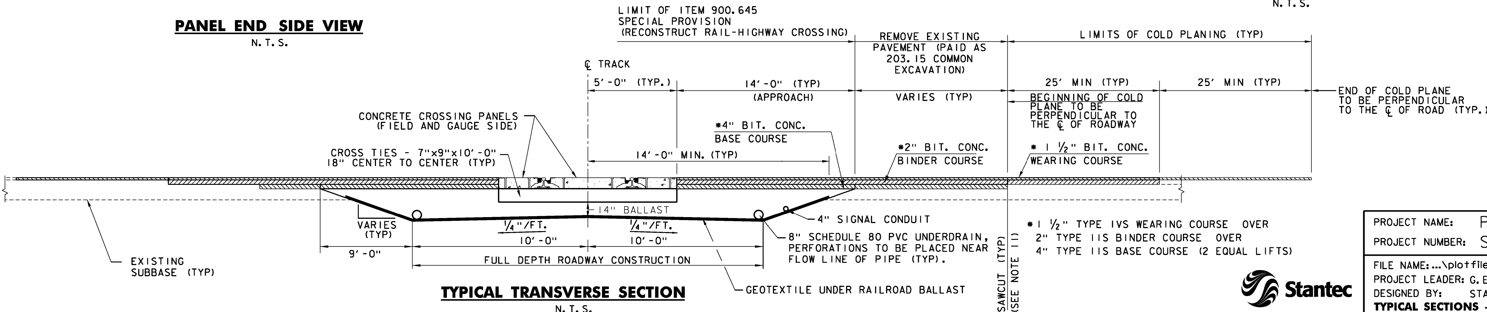
RAIL-SEALS TYPICAL SECTION N. T. S.
