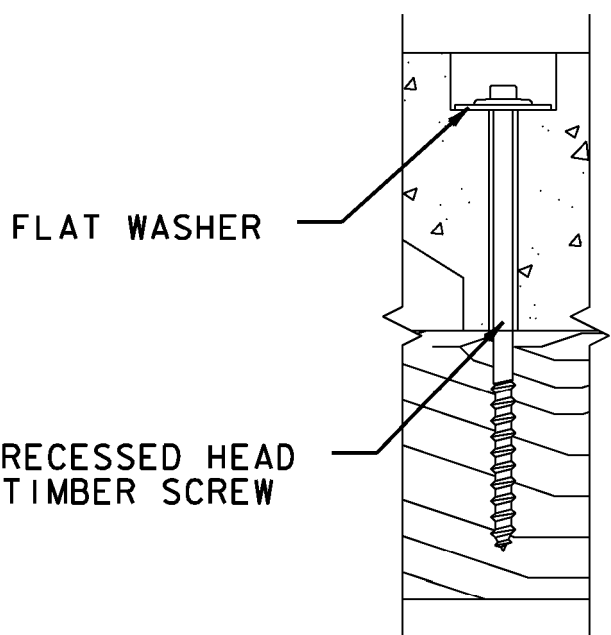
SCREW DETAIL N. T. S.
