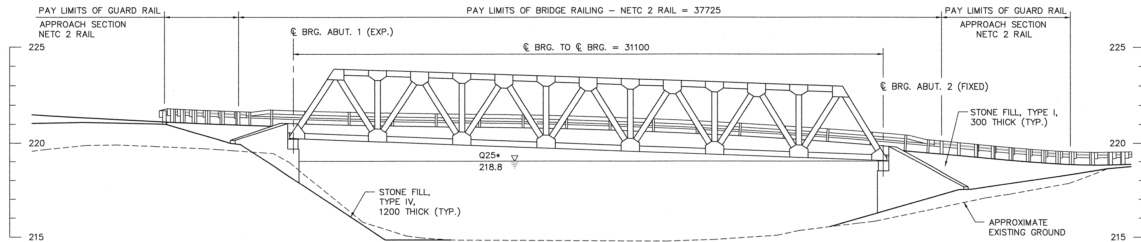
ELEVATION SCALE: 1:100
