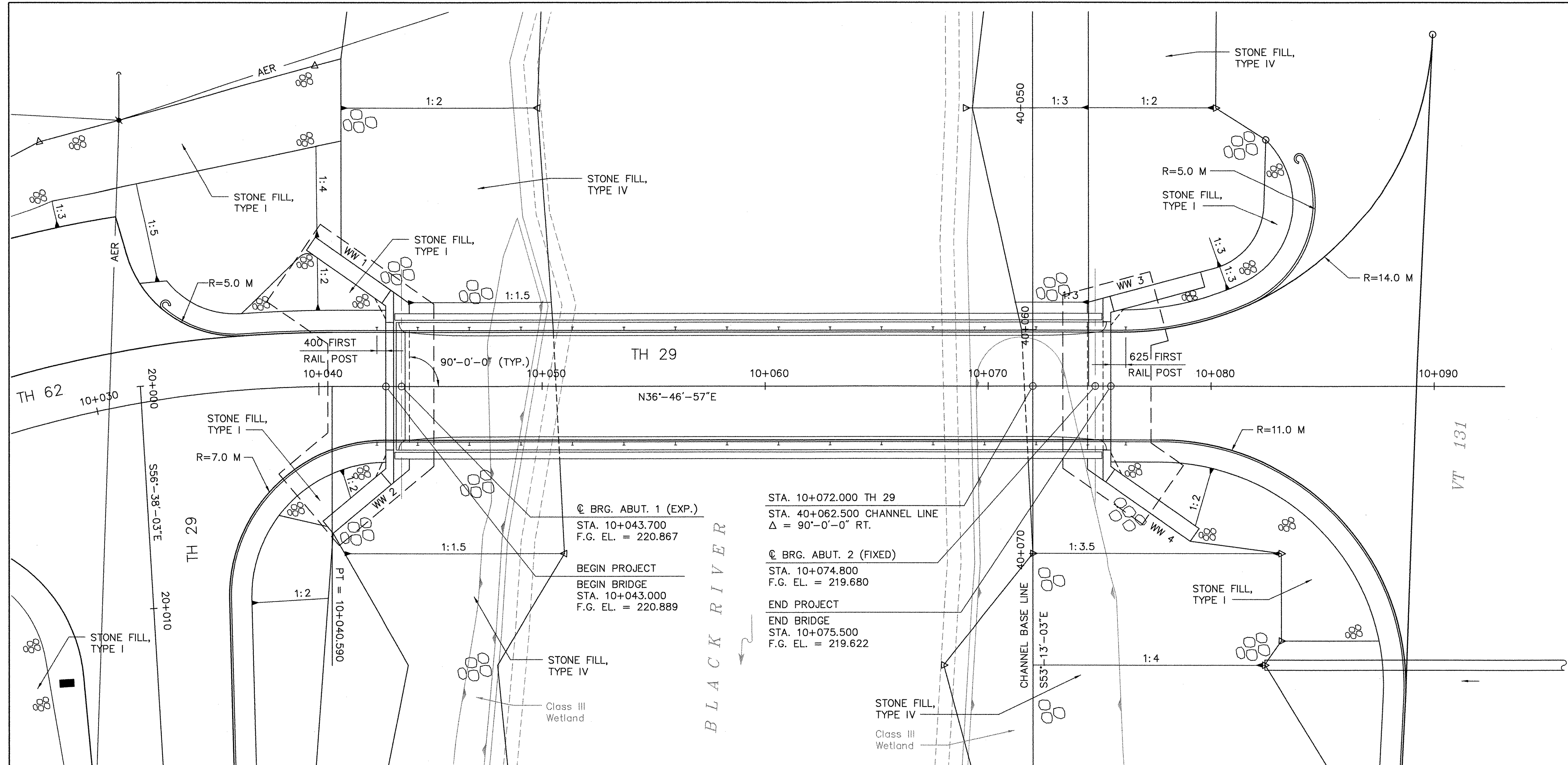
PLAN SCALE: 1:100
