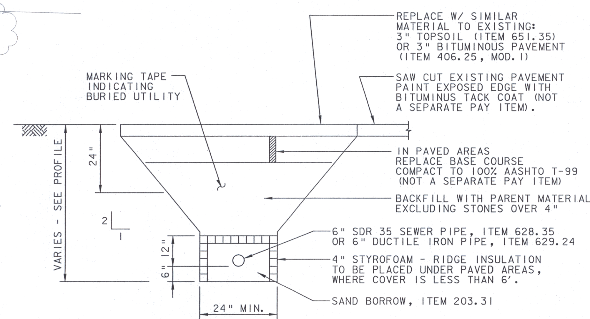
(D) 2 SEWERLINE TYPICAL SCALE: N. T. S.
