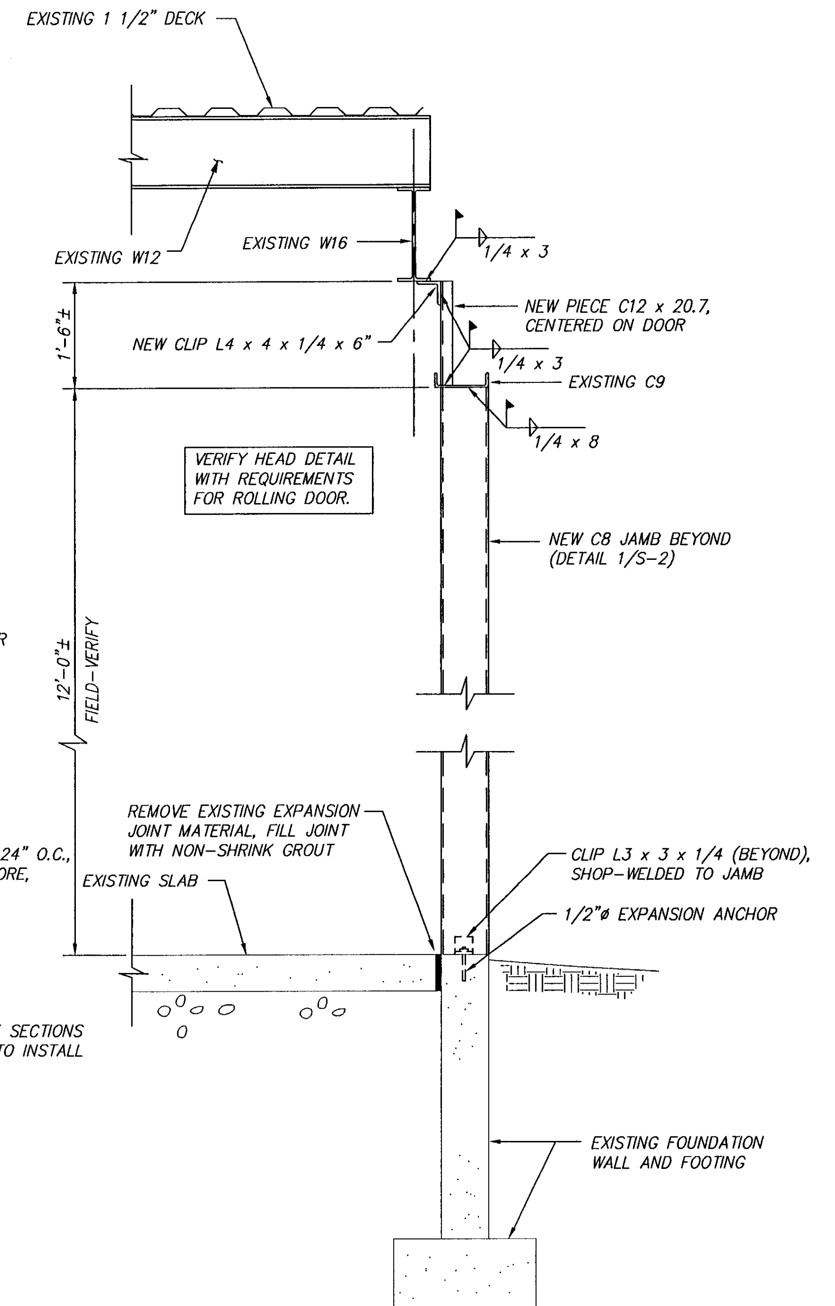
SECTION SCALE: 3/4" = 1'-0" (A S-2)
