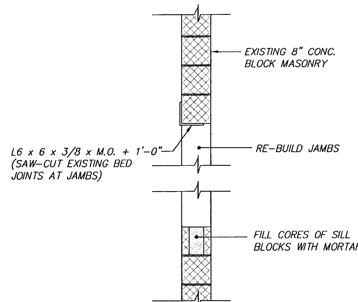
SECTION SCALE: 1 1/2" = 1'-0" (B S-2)
