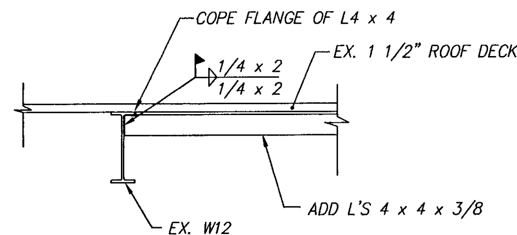
SECTION SCALE: 3/4" = 1'-0" (D S-2)
