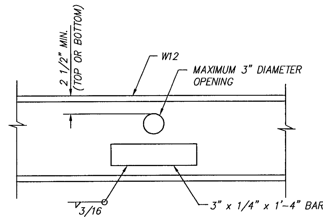
SECTION SCALE: 1 1/2" = 1'-0" (3 S-2)
