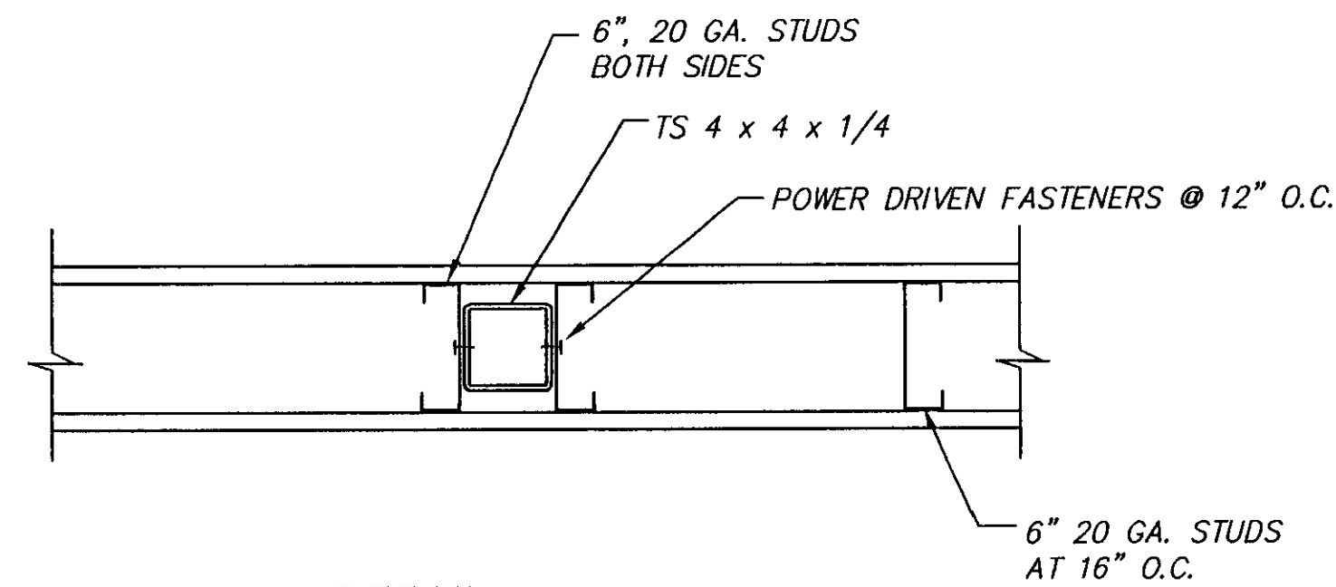
DETAIL SCALE: 1 1/2" = 1'-0" (2 S-2)
