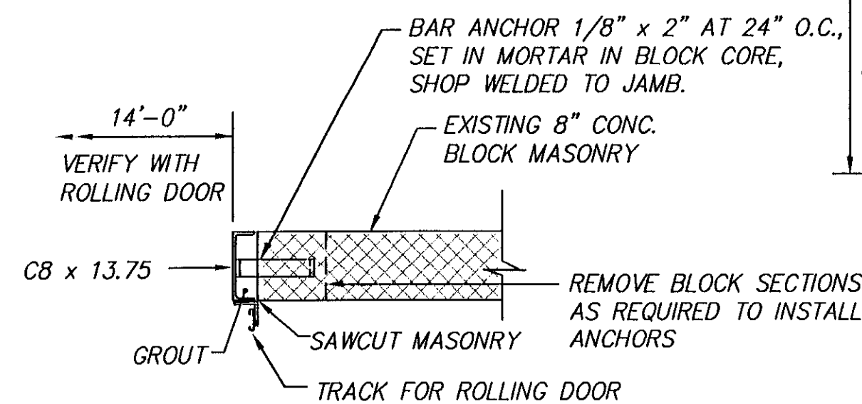
DETAIL SCALE: 3/4" = 1'-0" (1 S-2)
