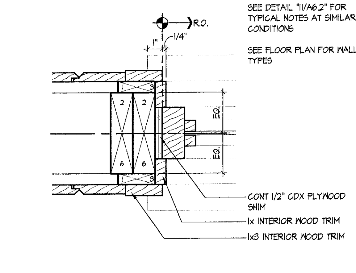
18 INTERIOR WINDOW JAMB SCALE: 3" = 1'-0"
