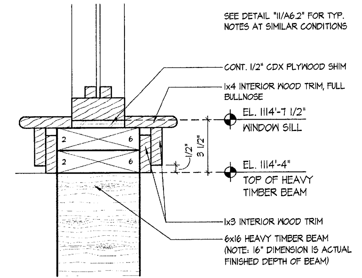
13 INTERIOR WINDOW SILL SCALE: 3" = 1'-0"
