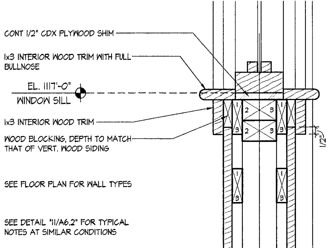
15 INTERIOR WINDOW SILL SCALE: 3" = 1'-0"
