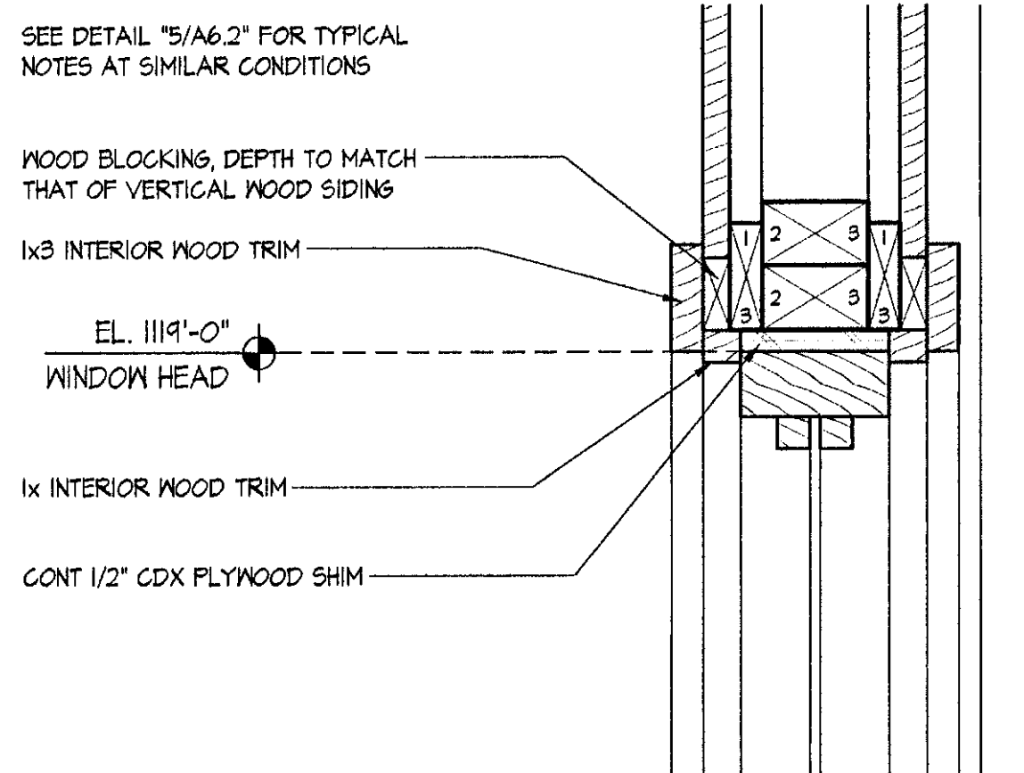
14 INTERIOR WINDOW HEAD/JAMB SIM. SCALE: 3" = 1'-0"
