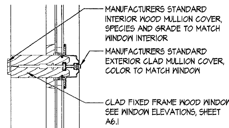
20 TYP. HORIZONTAL MULLION SCALE: 3" = 1'-0"
