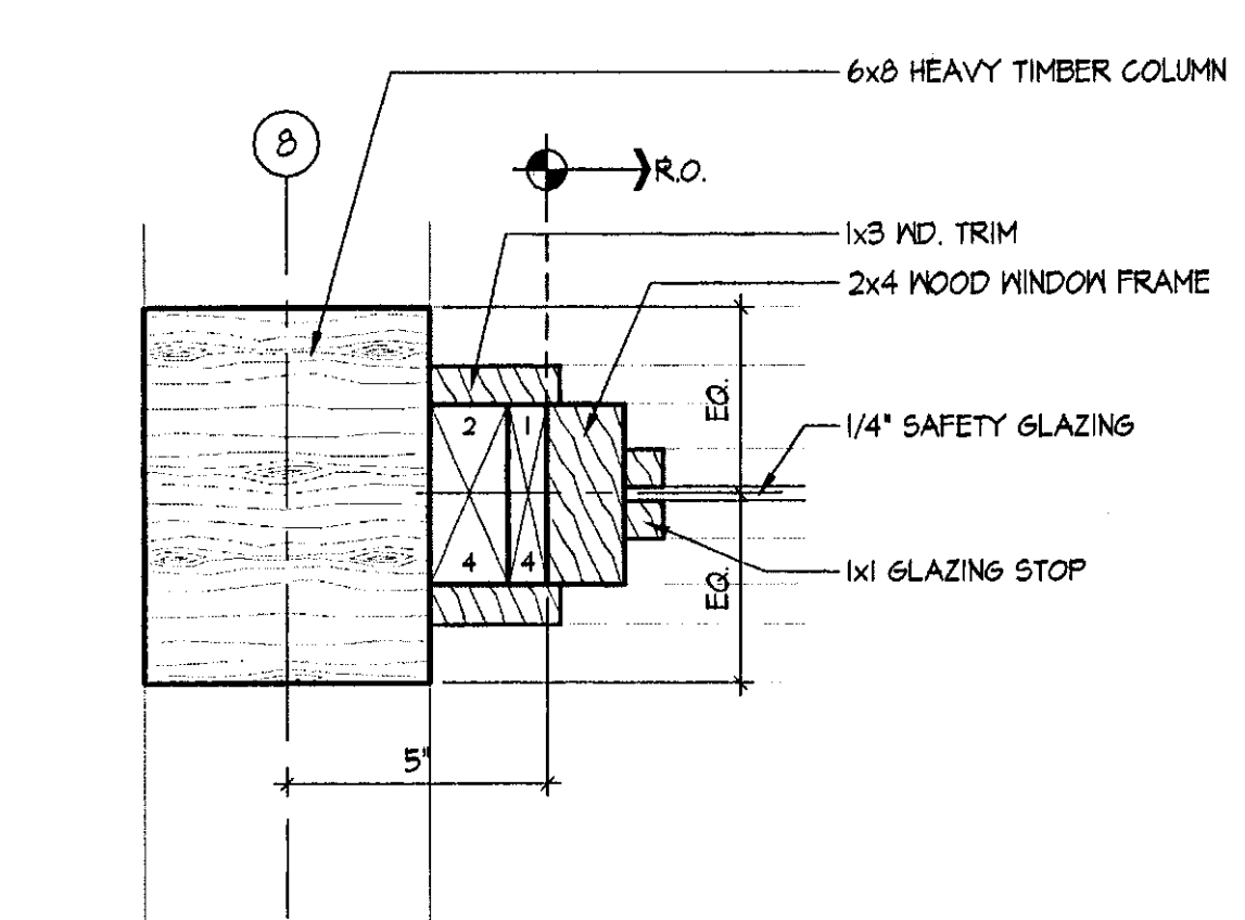
11 INTERIOR WINDOW JAMB SCALE: 3" = 1'-0"
