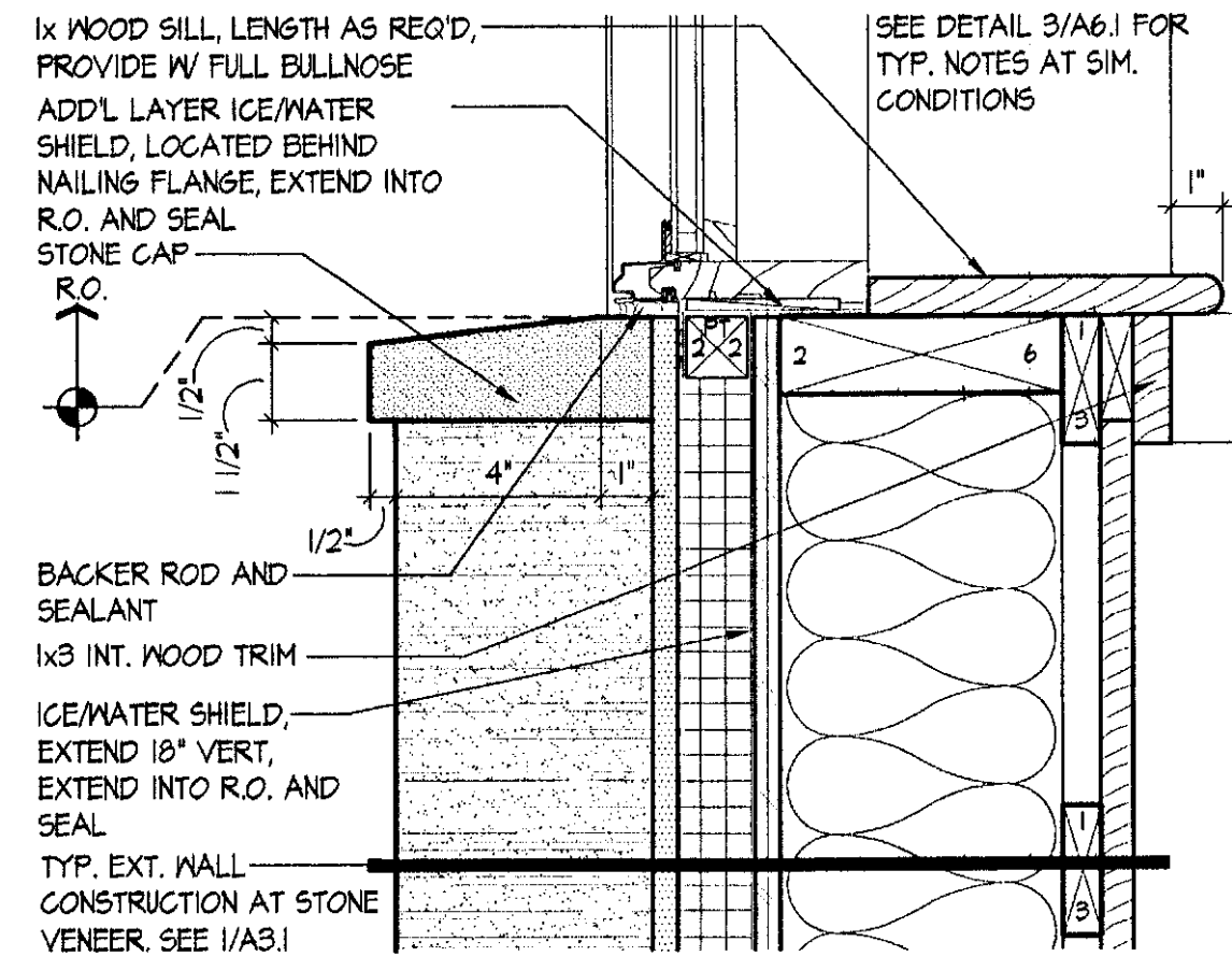
4 CLAD FRAME SILL @ STONE SCALE: 3" = 1'-0"
