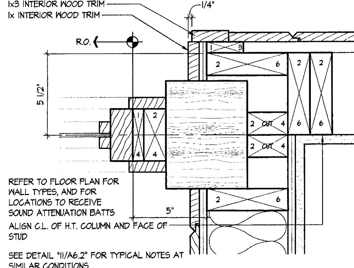
16 INTERIOR WINDOW JAMB SCALE: 3" = 1'-0"
