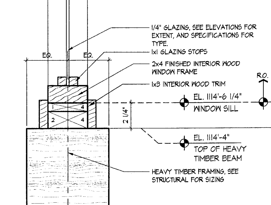
17 INTERIOR WINDOW SILL SCALE: 3" = 1'-0"
